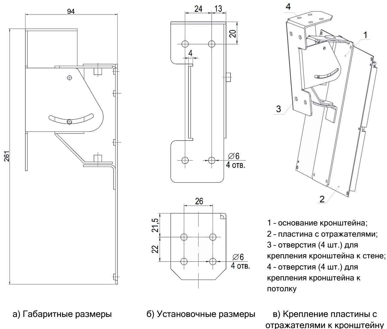
Рисунок 1 - Общий вид кронштейна
